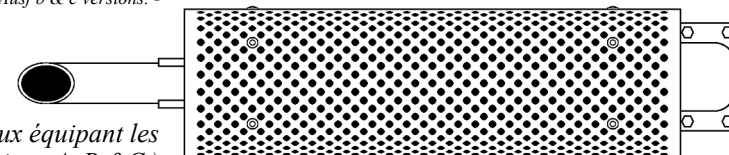
(Silencieux équipé de sa grille de protection sur les versions Ausf b & c.) - Muffler with protective grille on Ausf b & c versions. -
