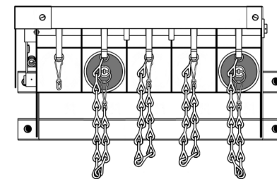
(Variante découpée pour recevoir les premiers modèles de nebelkerzenabwurfvorrichtung.) - Variant cut to accommodate the first models of nebelkerzenabwurfvorrichtung. -
