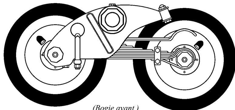
(Bogie avant.) - Front-Bogie avant.)
