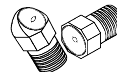
(Graisseurs plat & incliné.) - Flat and inclined grease nipple. -
