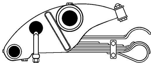
(bogie central et arrière.) - Central and rear bogie. -
