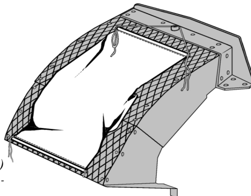
(Capot avant de garde-boue Ausf C.) - Mudguard front bonnet Ausf C. -
