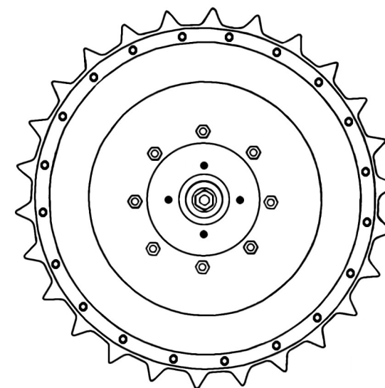
(Barbotin nu sans protection d'écrous.) - Bare sprocket without nut protection. -
